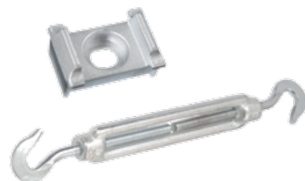
Alu-Auflageböcke und Schraubspanner sorgen für eine hohe Stabilität.
