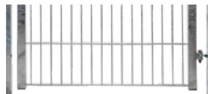
Die Torfüllung entspricht einer Doppelstabmatte vom Typ 8/6/8 und sorgt für eine tolle Optik.
