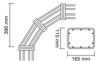
Eckelement 90° – Rechteck 115 / 165 mm
